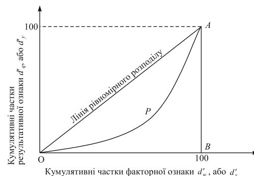
Рис. 1. Крива Лоренца
